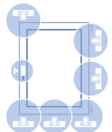
Fenster nachgerüstet mit einbruchhemmenden Beschlägen
